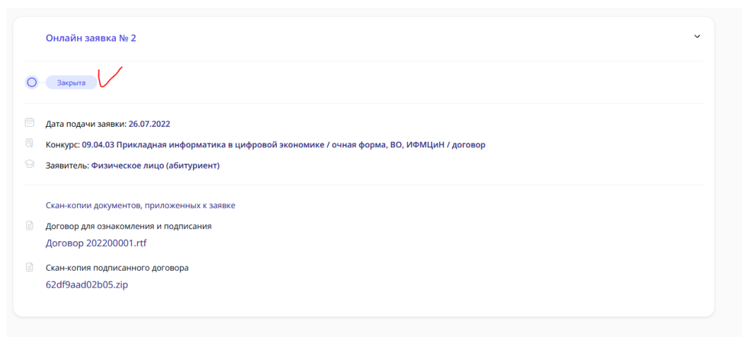
Рисунок 24 – Заявка закрыта.
